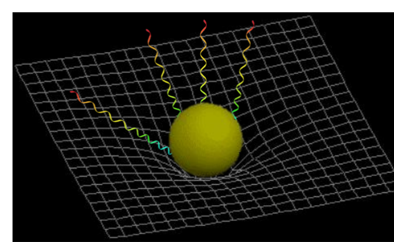
(그림8) 중력적색이동
